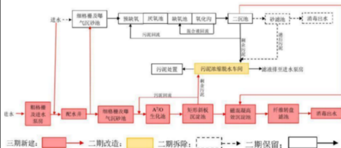
图3. 荷塘污水处理厂处理工艺流程图
